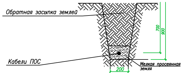
Траншея Т-1
