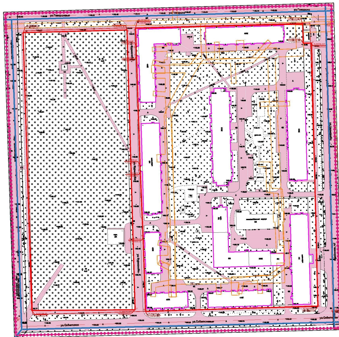
Схема красных линий и разбивочный чертеж красных линий. М 1:1000
