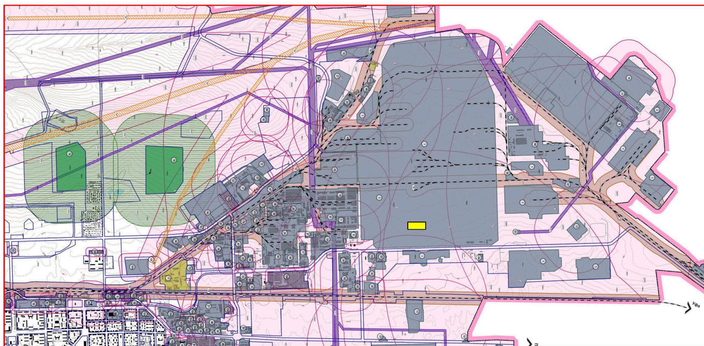
Схема границ зон с особыми условиями использования территории М1:20000
