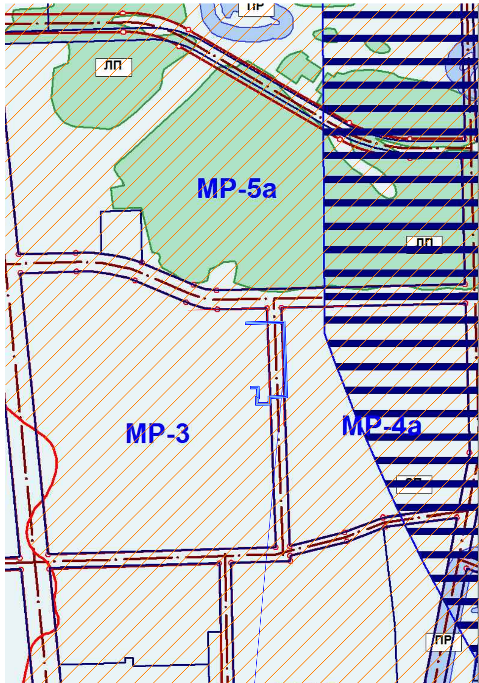
СХЕМА ГРАНИЦЫ ЗОН ПО ПРИРОДНО-ЭКОЛОГИЧЕСКИМ ТРЕБОВАНИЯМ
