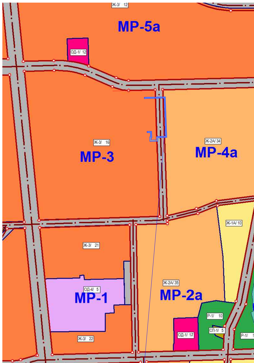
СХЕМА ГРАНИЦЫ ЗОН ГРАДОСТРОИТЕЛЬНОГО ЗОНИРОВАНИЯ
